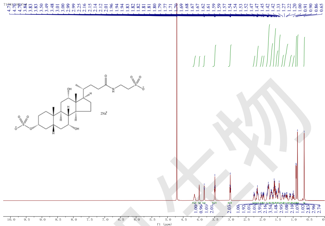
附图二 ( ^1\text{H-NMR} ):
